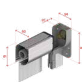
Piastra, testata e cassonetto da 50 mm
