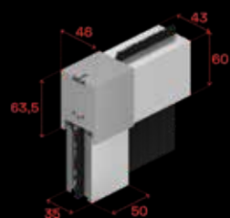
Cassonetto, cuffia e binario superiore
