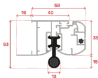
Telaio a Z, anta e cerniera standard
