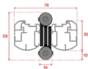
Telaio "Saloon", anta e cerniera "Saloon"
