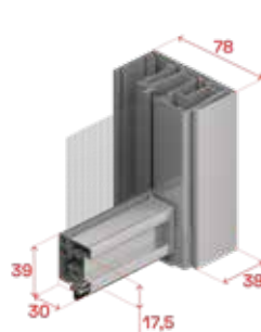
Distanziatore da 78, frontale, guida e maniglia
