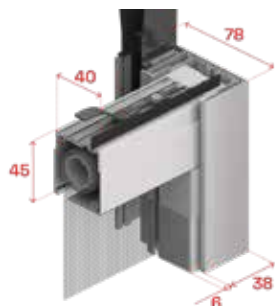
Distanziatore da 78, frontale, cassonetto, guida e maniglia
