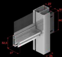
Maniglia, frontale guida e inserto di montaggio
