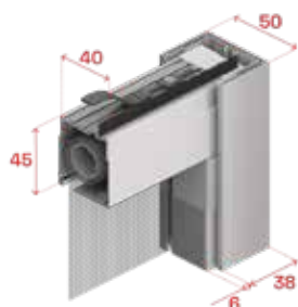
Distanziatore da 50, frontale, cassonetto, guida e maniglia
