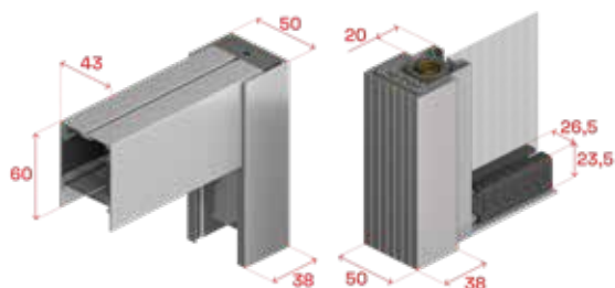
Distanziatore da 50, frontale e binario superiore
