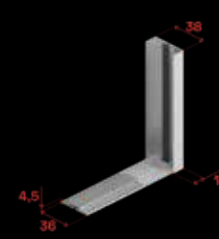
Binario inferiore e compensatore magnetico
