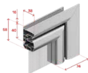
Telaio a Z
