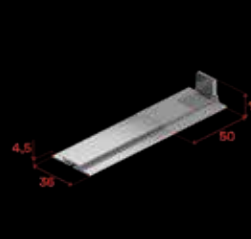
Binario inferiore e finecorsa con piastrina magnetica
