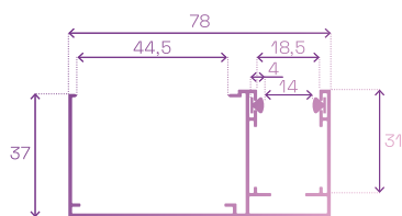
DISTANZIATORE da 78 mm
