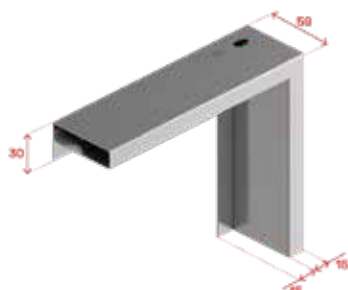
Telaio
