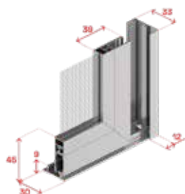
Pannello, binario inferiore e terminale
