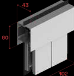
Cassonetti spalla a spalla e binario superiore
