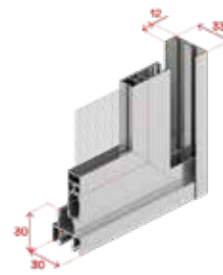
Binario inferiore alto, pannello e terminale
