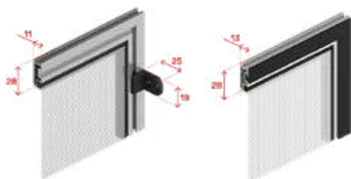
Profilo e angolare di fissaggio
