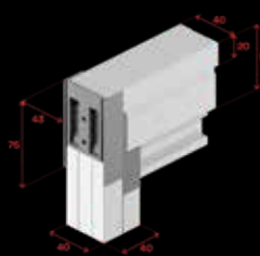
Compensatore superiore, compensatore, guida e cassonetto
