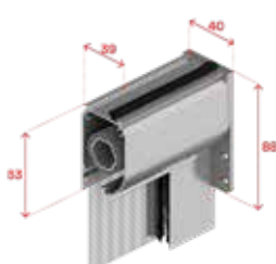
Piastra singola e cassonetto da 40 mm
