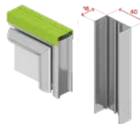
Compensatore
