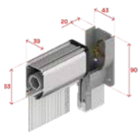
Piastra, testata e cassonetto da 40 mm
