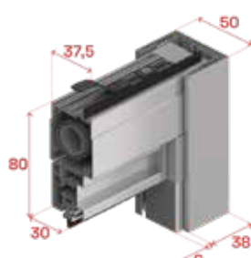
Distanziatore da 50, frontale, guida e maniglia
