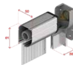
Piastra per guida alta, guida alta, testata e cassonetto da 50 mm
