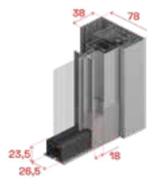
Distanziatore da 78, frontale, maniglia e catenaria
