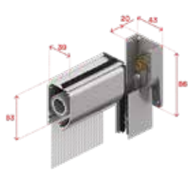
Piastra doppia, testata e cassonetto da 40 mm
