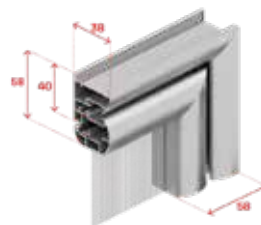
Telaio a L
