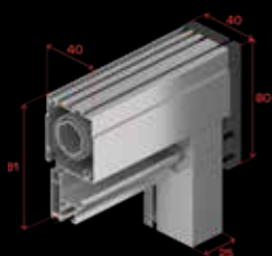
Cassonetto, cuffia, maniglia e frontale guida
