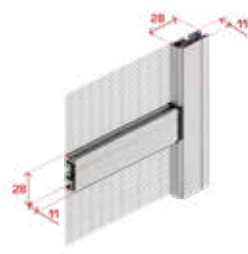
Traversa
