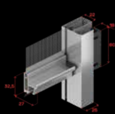
Frontale guida, maniglia con scivolo sagomato e inserto di montaggio
