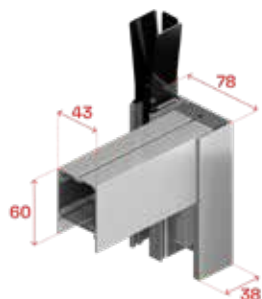
Distanziatore da 78, frontale e binario superiore
