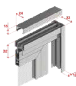
Binario superiore, compensatore, pannello e terminale
