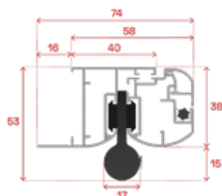
Telaio a Z, anta e cerniera con molla di ritorno
