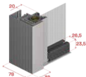
Distanziatore da 78, frontale, cassonetto e catenaria
