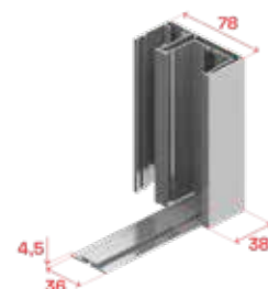
Distanziatore da 78, frontale e binario inferiore con finecorsa
