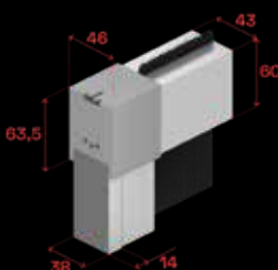
Compensatore, cuffia e binario superiore
