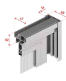
Binario superiore a 3 vie, compensatore e terminale
