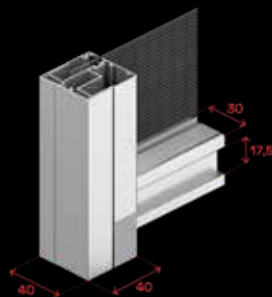
Compensatore, guida e maniglia
