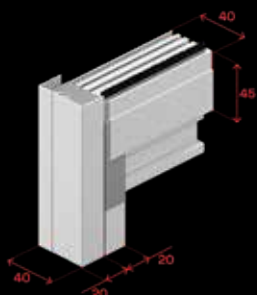
Compensatore, guida, cassonetto e maniglia
