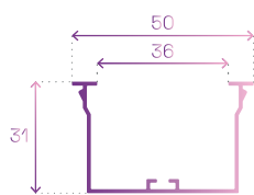
FRONTALE ISW5 CASSONETTO/TERMINALE
