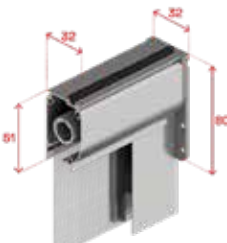
Piastra singola e cassonetto da 32 mm
