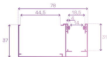
DISTANZIATORE da 78 mm
