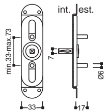
Movimento Gratz Q7 con perni 10 15
