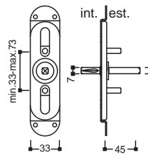
Movimento Gratz Q7 +7 con perni 10 16
