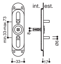
Movimento Gratz Q8 con perni 10 17
