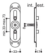
Movimento Gratz Q8 con fori 10 22
