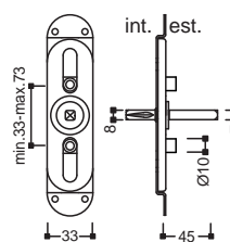
Movimento Gratz Q8 +7 con fori 10 23
