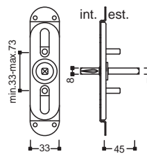
Movimento Gratz Q8 +7 con perni 10 18
