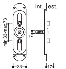
Movimento Gratz Q7 con fori 10 20
