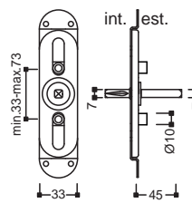
Movimento Gratz Q7 +7 con fori 10 21
