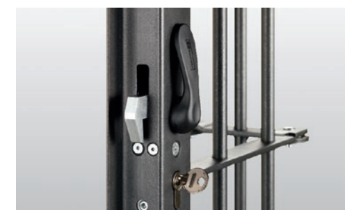
Maniglia ad ingombro ridotto e cilindro ribassato
